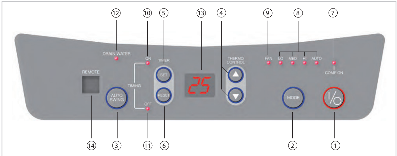
Obr. 3: Ovládací panel
