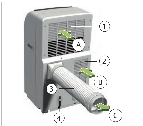
Obr. 2: Pohled zezadu
