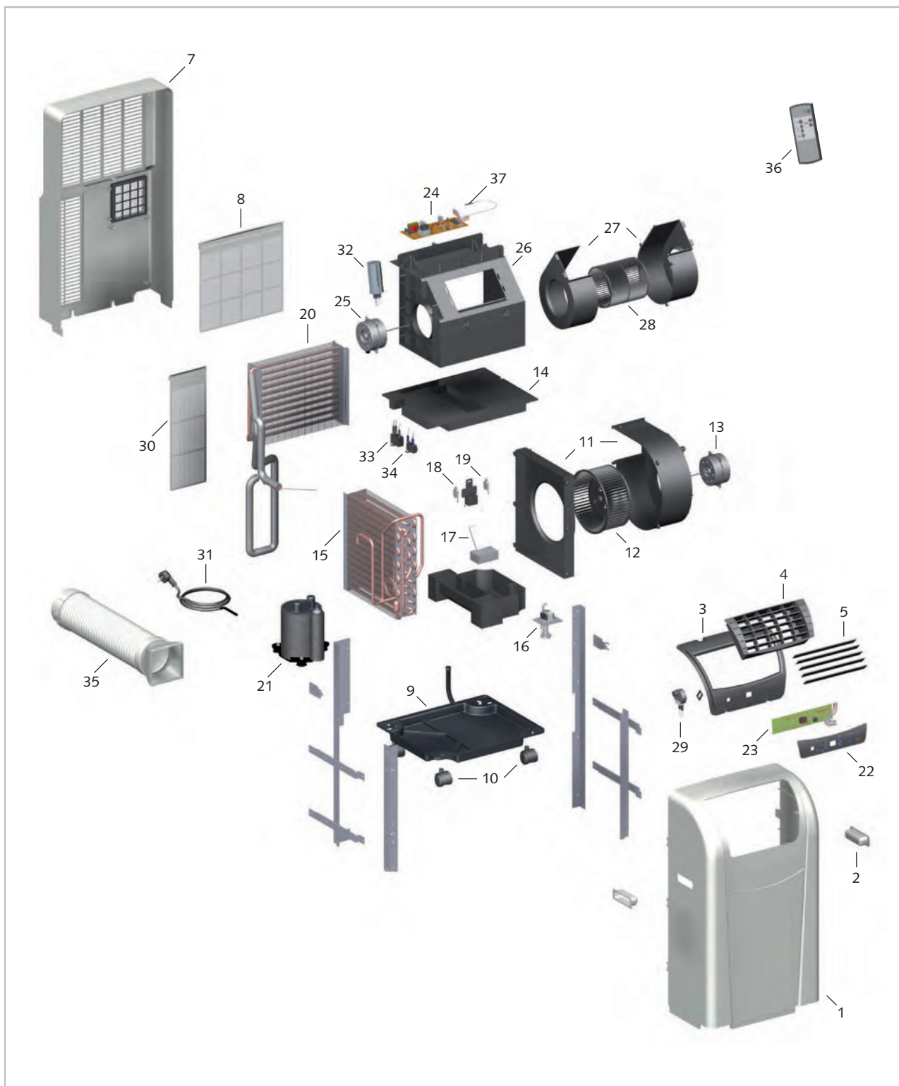
Obr. 16: Explozivní výkres
